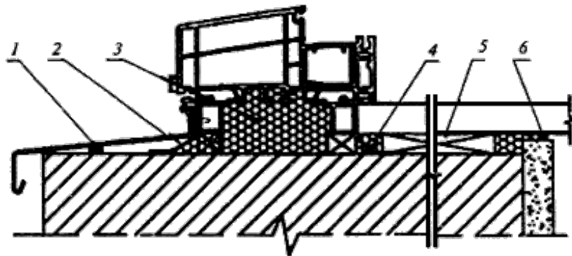
Рисунок А.11 - Монтажный шов в нижнем узле примыкания коробки балконной двери
