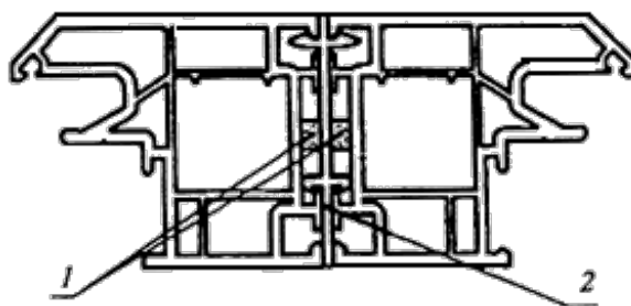
Рисунок А.14 - Монтажный шов узла примыкания оконного блока к стеновому проему с отделкой наружного откоса и фасада паропроницаемым штукатурным раствором
