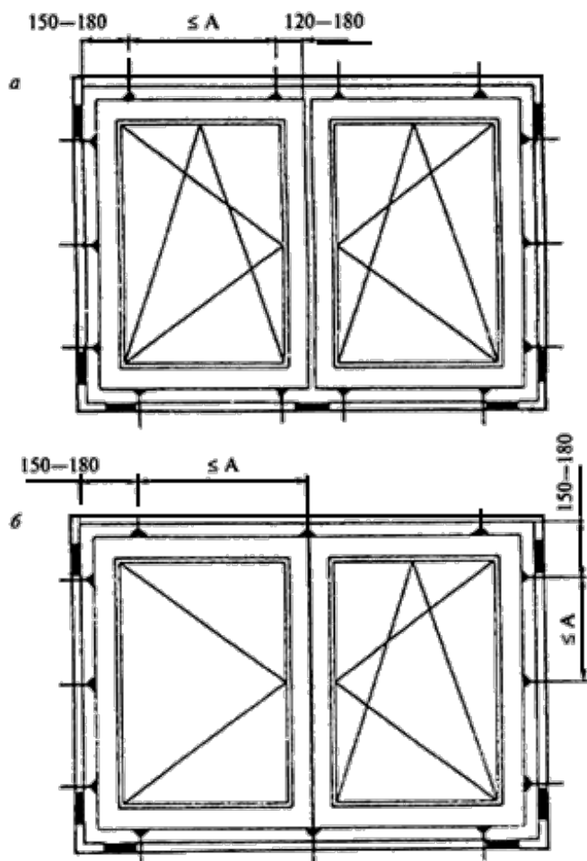
а - оконный блок с вертикальным импостом; б - оконный блок с безимпостным (штульповым) притвором;
