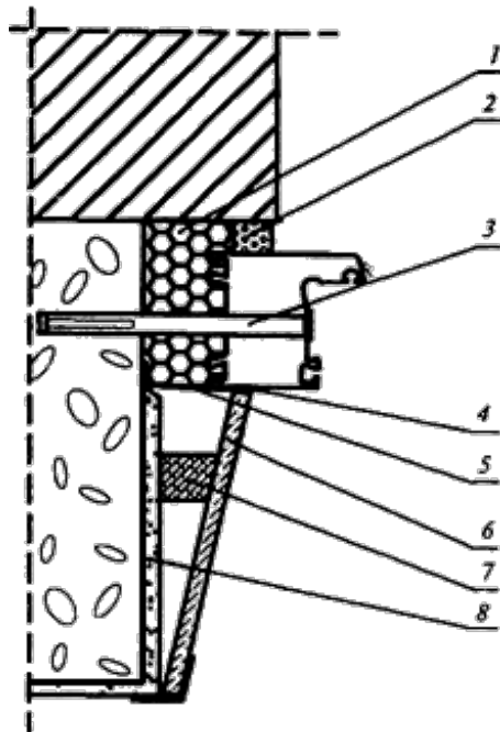
Рисунок А.5 - Узел верхнего примыкания оконного блока к перемычке из стального уголка в проеме многослойной стены с облицовкой кирпичом
