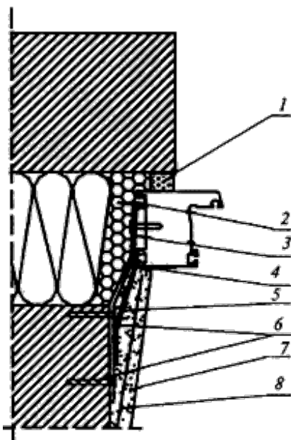
Рисунок А.2 - Узел бокового примыкания оконного блока к проему без четверти в стене из кирпича и отделкой внутреннего откоса облицовочной панелью
